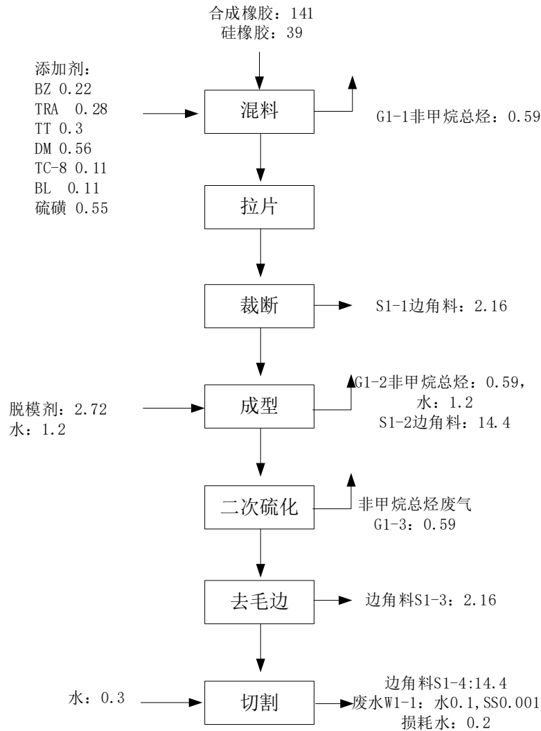
图 3.5-1 合成橡胶滚轴和硅橡胶滚轴生产工艺及产污环节流程图
