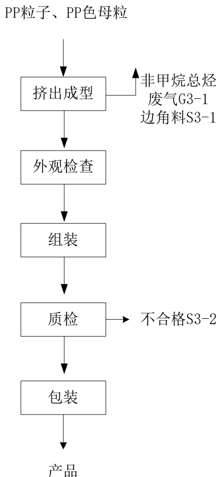
图 3.5-2 汽车内饰配件生产工艺及产污环节流程图
