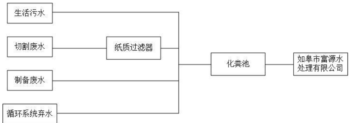
图4.1-1 废水治理工艺流程图
